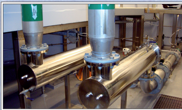
UV-behandling i Lekaryd för vatten till Alvesta.
